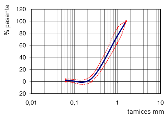
Análisis granulométrico (UNE-EN 933-1)
