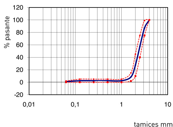
Análisis granulométrico (UNE-EN 933-1)
