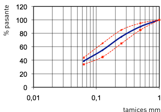
Análisis granulométrico (UNE-EN 933-1)
